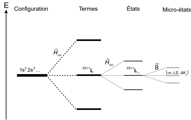
FIGURE 41 – Perturbations successives dans le cadre du couplage de Russel-Saunders (inspiré de “Introduction à la chimie quantique” de Claude Leforestier).
