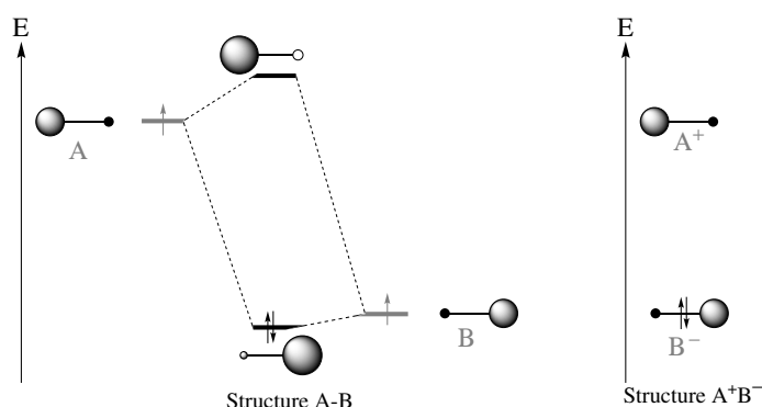
FIGURE 20 – Interaction entre deux atomes aux électronégativités très différentes.
