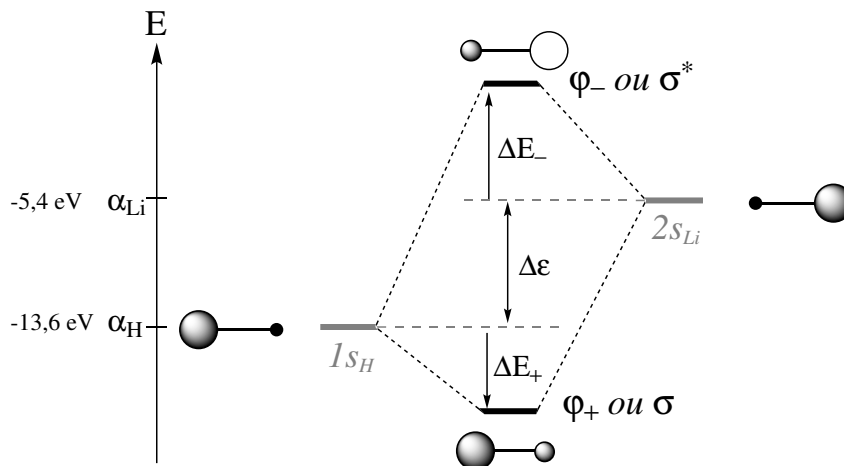
FIGURE 19 – Diagramme d'interaction de LiH.
