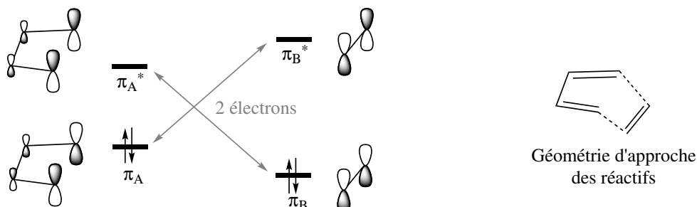
FIGURE 34 – Interactions entre OF au cours de la réaction de Diels-Alder.
