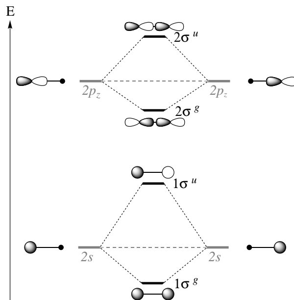
FIGURE 28 – OM de symétrie \sigma des molécules de dioxygène ou de difluor.
