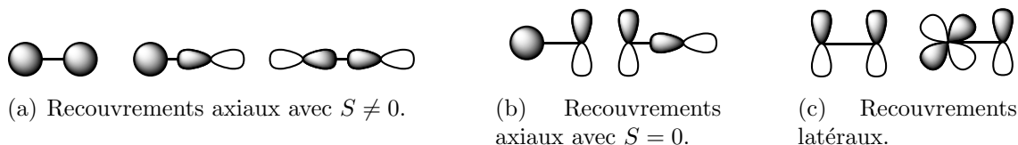
FIGURE 21 – Recouvrements possibles entre orbitales atomiques.
