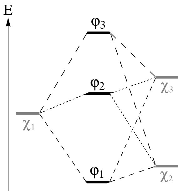
FIGURE 23 – Interaction à trois orbitales.
