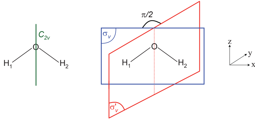
FIGURE 12 – Symétries de la molécule d'eau dans sa géométrie d'équilibre.
