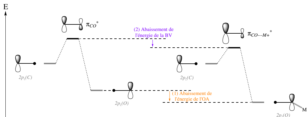
FIGURE 37 – Assistance électrophile d'un carbonyle par un cation métallique.
