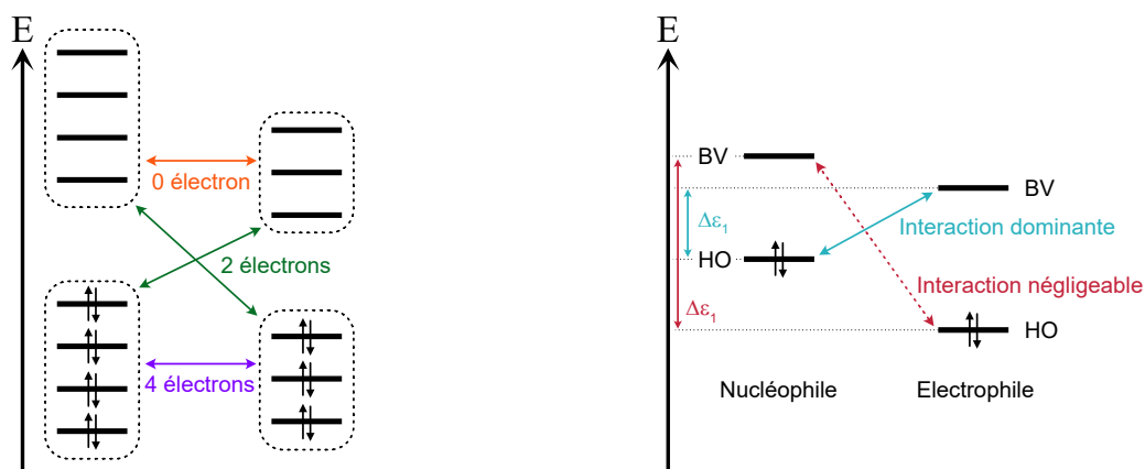
FIGURE 33 – Interactions entre orbitales, et illustration de la règle de Fukui.
