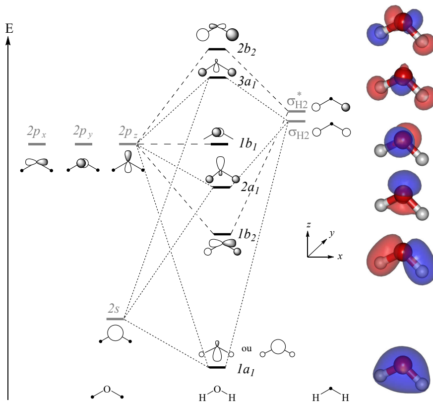
FIGURE 24 – Diagramme d'interaction entre les orbitales de O et celles de H_2 pour OH_2 coudée, et représentation des OM calculées.
