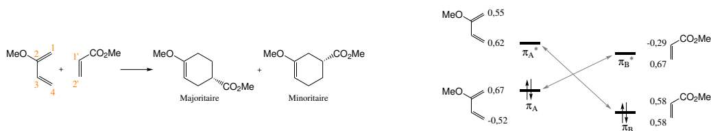
FIGURE 35 – Régiosélectivité de la réaction de Diels-Alder.
