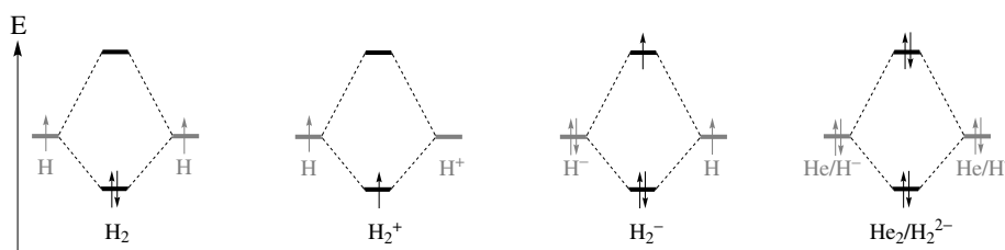
FIGURE 18 – Remplissage de quelques molécules diatomiques simples.
