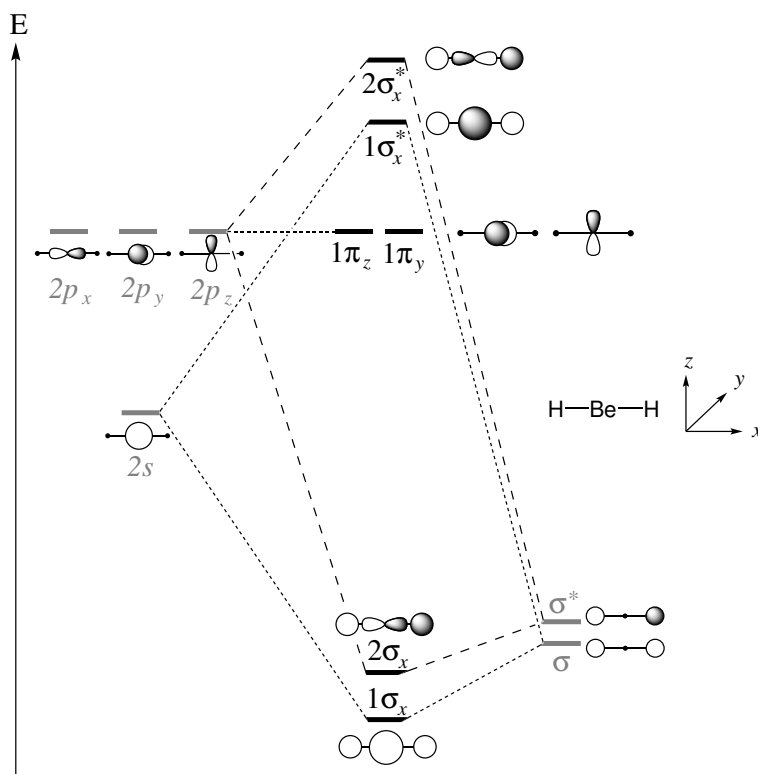
FIGURE 22 – Diagramme d'interaction entre Be et H_2 pour BeH_2 linéaire.
