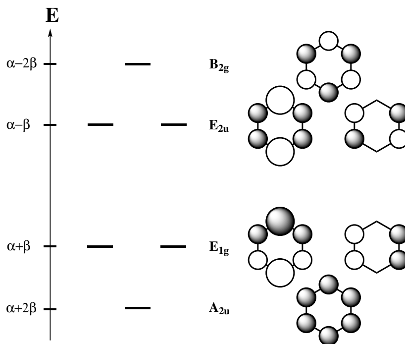
FIGURE 13 – Diagrammes d'OM de la molécule de benzène.
