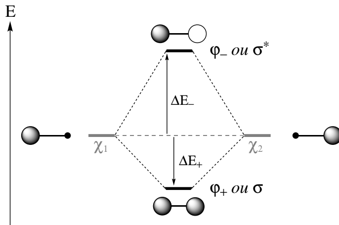
FIGURE 17 – Diagramme énergétique des OM de H_2 .
