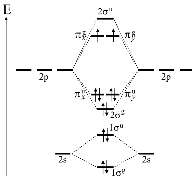
FIGURE 29 – Diagramme d'OM des molécules de dioxygène ou de difluor.
