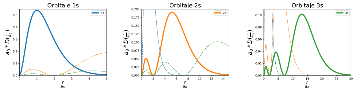
FIGURE 6 – Densités de probabilité de présence d'un électron ns pour l'hydrogène. Sur chaque panel, les densités des trois OA sont représentées pour comparaison.
