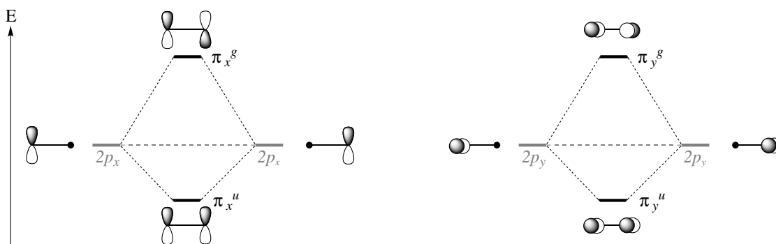
FIGURE 27 – OM de symétrie \pi des molécules de dioxygène ou de difluor.
