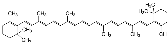
FIGURE 39 – Structure du carotène.
