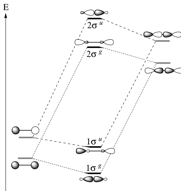
FIGURE 30 – OM de symétrie \sigma de la molécule de diazote.
