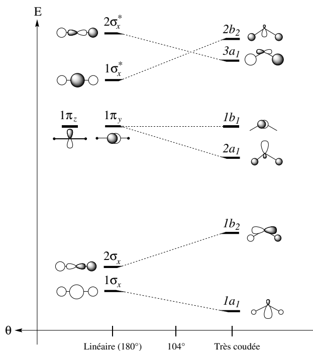
FIGURE 26 – Diagramme de Walsh selon l'angle pour les molécules AH_2 .
