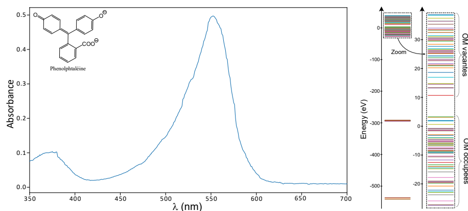
FIGURE 38 – Spectre d'absorption de la phénolphtaléine et diagramme d'OM (les niveaux énergétiques ne sont qu'approximatifs en raison de la méthode de calcul).
