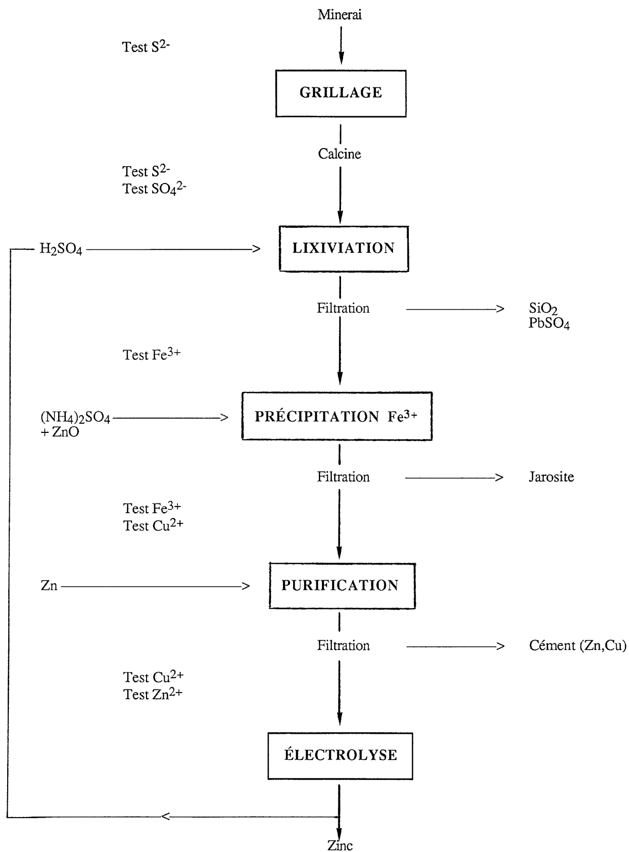
Figure 1 : Schéma des opérations hydrométallurgiques, au laboratoire.
