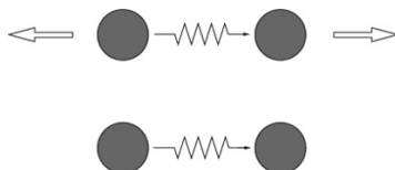
Fig. VIII.9. L'effet Mössbauer en images : le schéma du haut montre le recul d'un noyau libre (à gauche en émission et à droite en absorption de rayon gamma). Dans le schéma du bas, l'absorption ou l'émission se produisent sans recul, comme si la masse du noyau était infinie. Si les noyaux émetteur et récepteur sont dans un environnement cristallin identique, l'énergie des transitions radiatives sont exactement les mêmes ; émission et absorption sont des phénomènes résonants.
