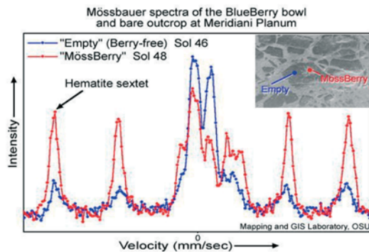
Fig. VIII.12. Spectres Mössbauer du fond de la roche et de l'accumulation de myrtilles. Les spectres ont été enregistrés, respectivement, le 46 me et 48 me jours martiens de la mission ( sol ), pour le bol vide et le bol plein. Source : NASA/JPL/Cornell/University of Mainz.
