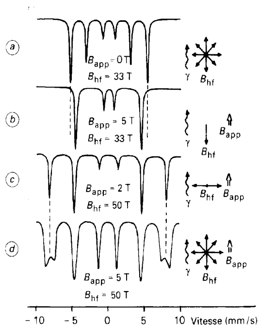
Fig. VIII.6. Spectres Mössbauer de ^{57}\text{Fe} dans différents matériaux magnétiques. (a) Matériau polycristallin ferromagnétique ( B_{app} = 0\text{ T} ), (b) matériau polycristallin ferromagnétique saturé par une induction appliquée parallèlement au faisceau \gamma ( \mathbf{B}_{hf} et \mathbf{B}_{app} de sens opposés), (c) matériau polycristallin antiferromagnétique à l'équilibre, les moments magnétiques sont perpendiculaires à \mathbf{B}_{app} , (d) matériau dont les directions des moments magnétiques ne sont pas affectées par l'induction extérieure.
