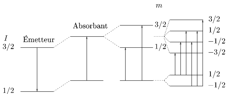
Fig. VIII.3. Déplacement des niveaux nucléaires sous l'action des interactions hyperfines dans le cas d'une transition entre des états de spin 3/2 et 1/2 .
